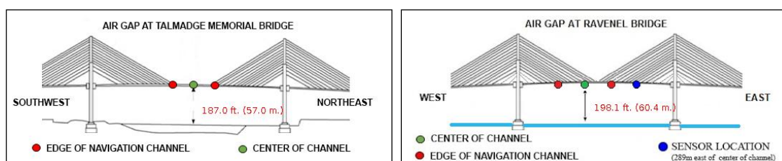
Slika 42. Općeniti prikaz preostale visine iznad vode za mostove Talamadge memorial i Ravel, Izvor NOAA 285
