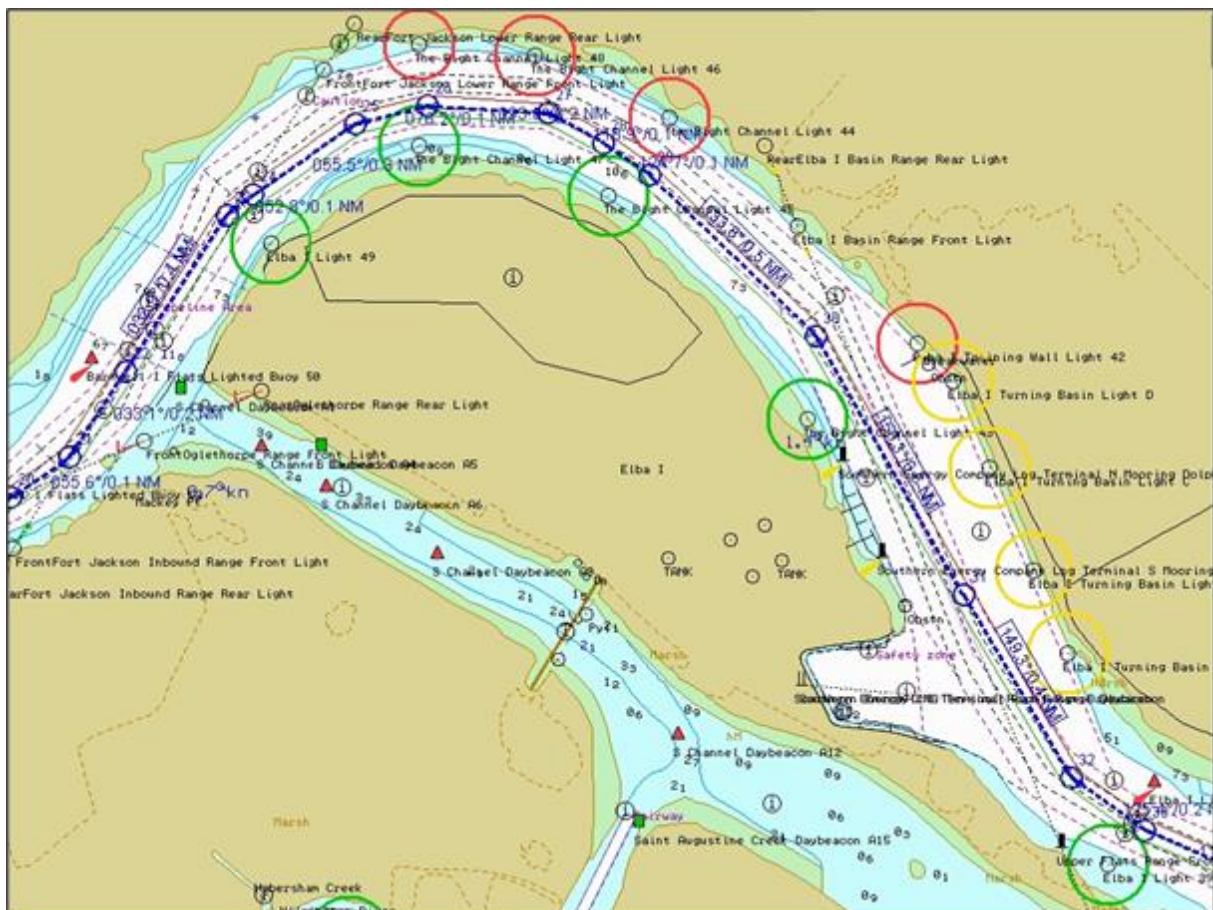
Slika 68. Prikaz dobivenog puta u zavojitom dijelu prilaznoga plovnog puta luke Savannah. Priredio autor koristeći slikovne zapise NTPRO 5000 navigacijskog simulatora
