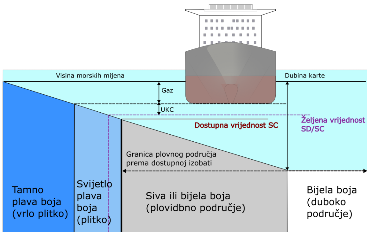
Slika 17. Prikaz izobate plitke vode, sigurne izobata i izobate duboke vode
