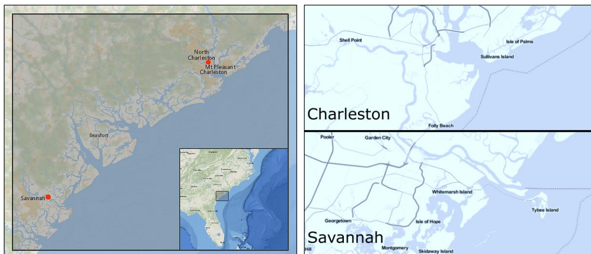
Slika 30. Odaabrano plovidbeno područje na istočnoj obali SAD-a između luka Savannah i Charleston (lijevo dolje). Zasjenjeni okvir prikazuje granice odabranog AIS područja i luke (lijevo). Neposredni prilaz lukama (desno). Priredio autor
