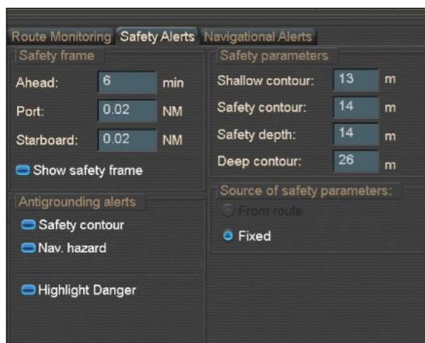
Slika 66. Prikaz osnovnih horizontalnih i vertikalnih ograničenja u ECDIS simulatoru.
